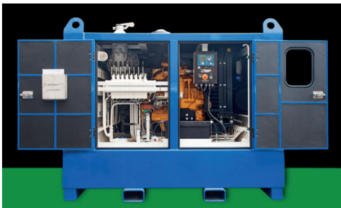
Hydraulische Antriebseinheit (HPU) / Hydraulic Power Unit (HPU)
