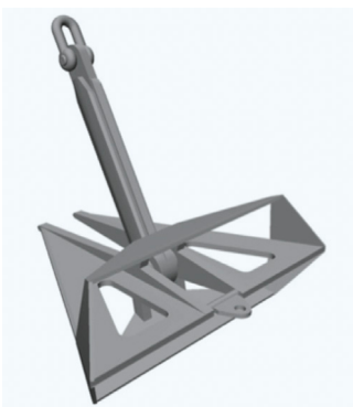
Anchor Delta Flipper 2000 kg auch als 5000 kg Anker vorhanden (4x)
